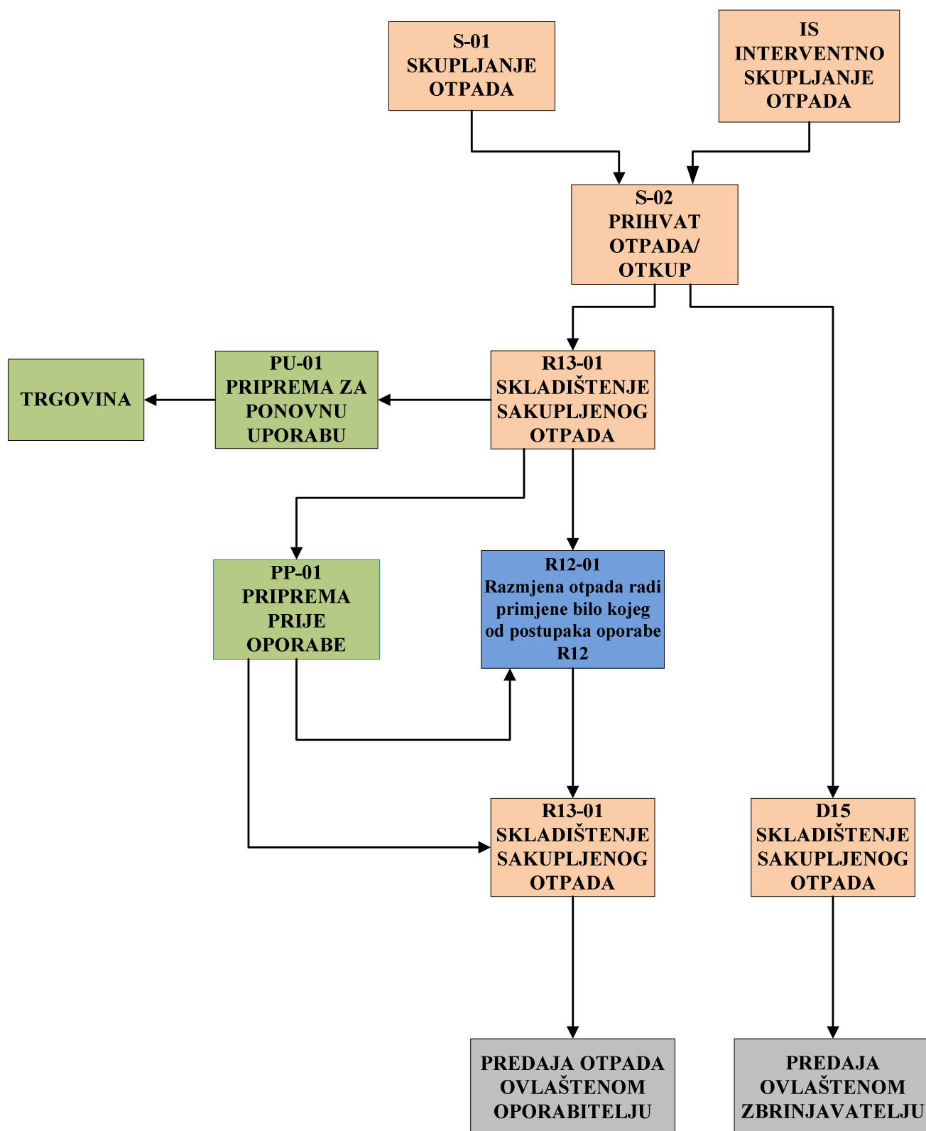
Slika 1. Shematski prikaz tehnoloških procesa
