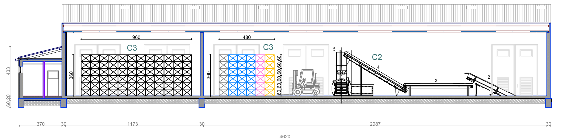
Pogled a-a
