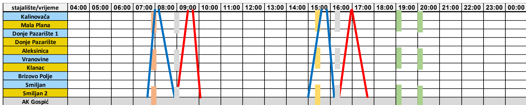
Grafikon 11: Prikaz grafikona predloženog voznog reda linije B
